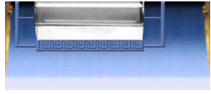
romain.bmp
